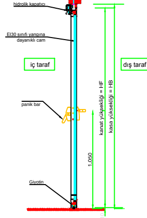
KESİT
