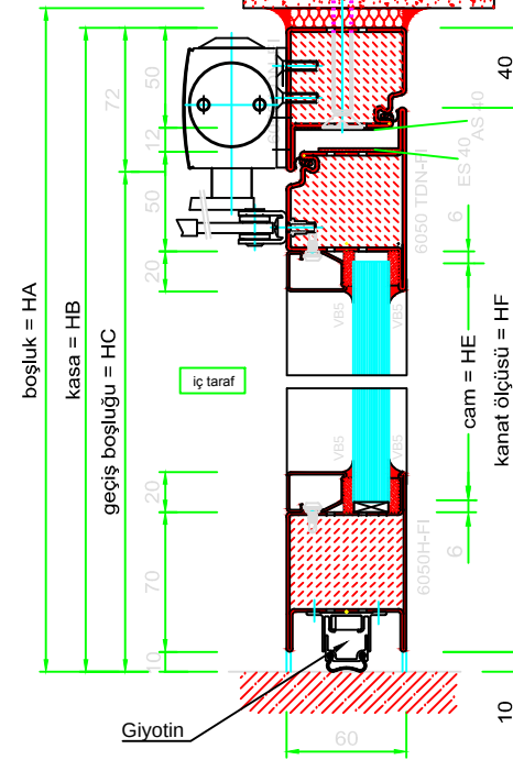
B-B KESİTİ
