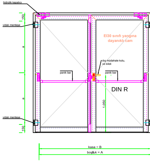
DİŞTAN GÖRÜNÜŞÜ
