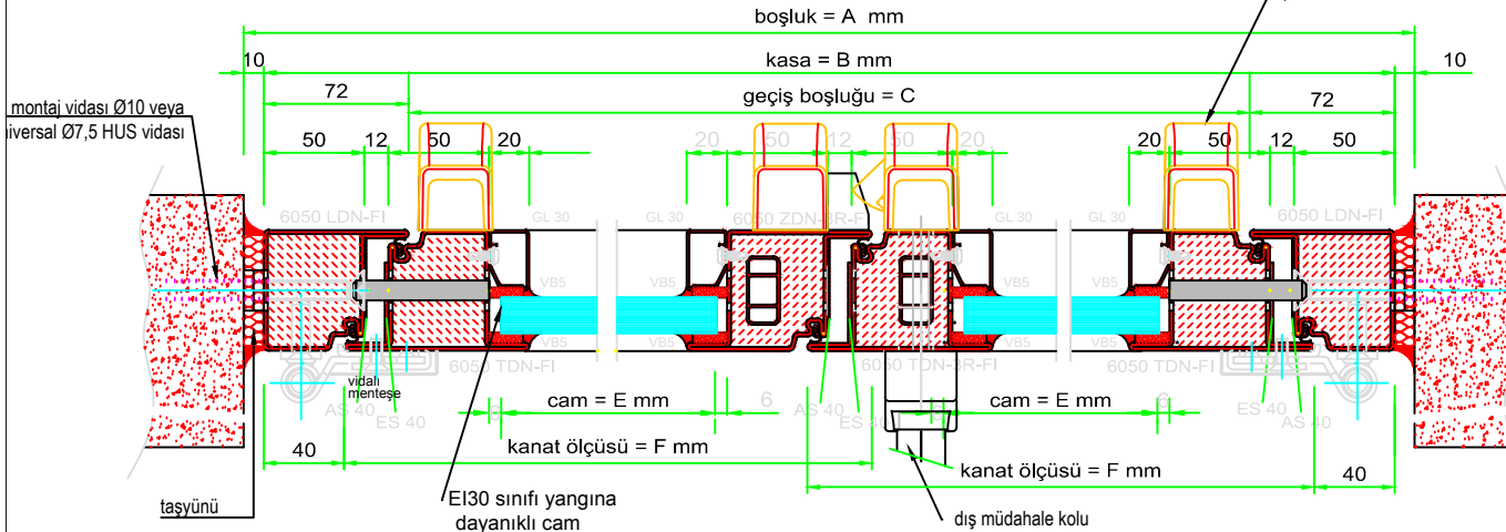
A-A KESİTİ
