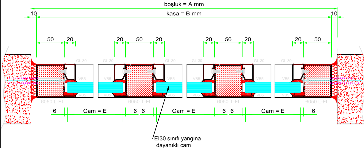
A-A KESİTİ
