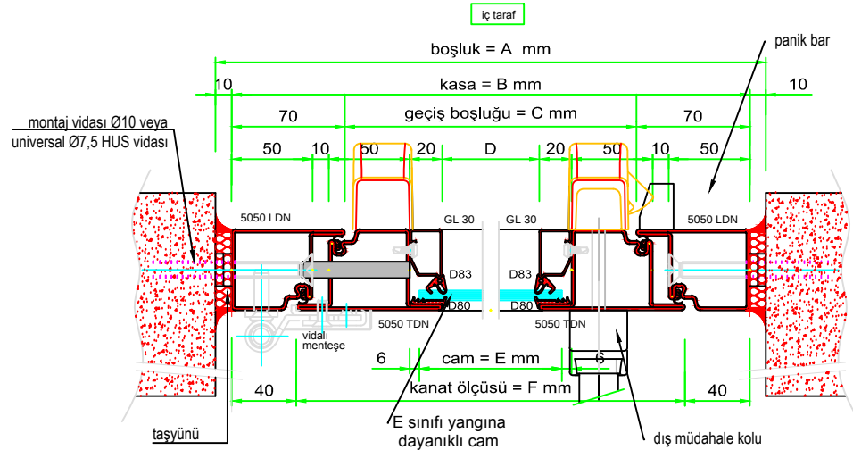
A-A KESİTİ
