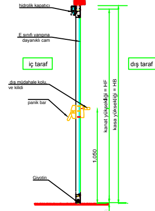
KESİT
