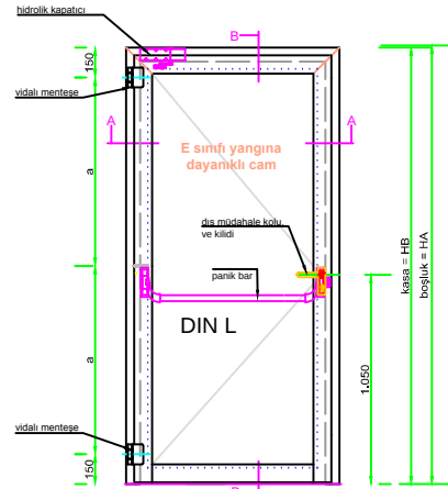
DIŞTAN GÖRÜNÜŞÜ
